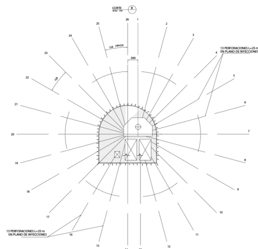
Corte B- Caverna de Válvulas Inyecciones.
