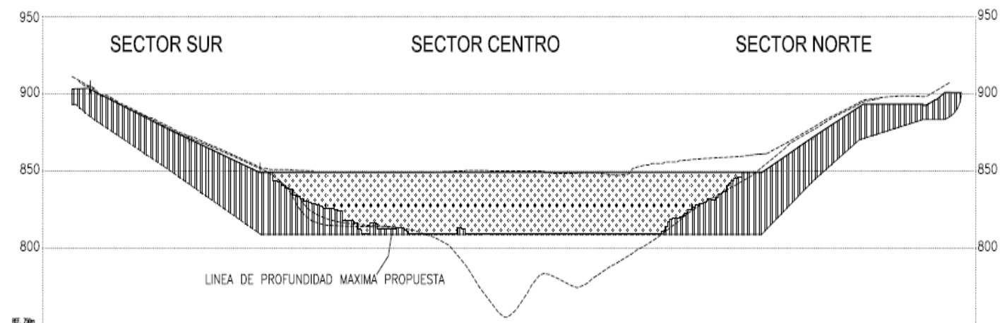
Perfil Longitudinal Inyecciones de Impermeabilización.
