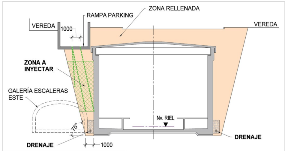
Figura 1 – Excavación línea 1 en trinchera.
