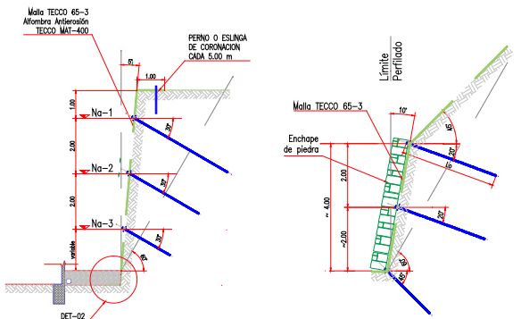
Instalación de los Anclajes Pasivos o Nails.
