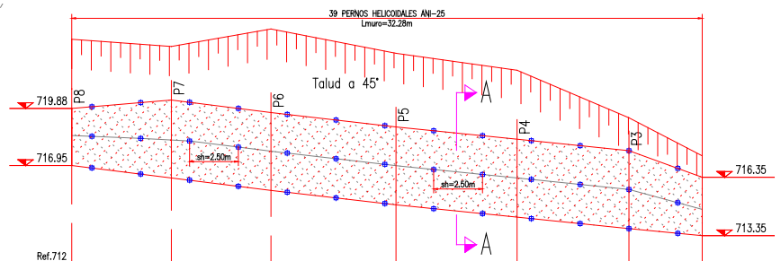
Cortes y Elevación muros.
